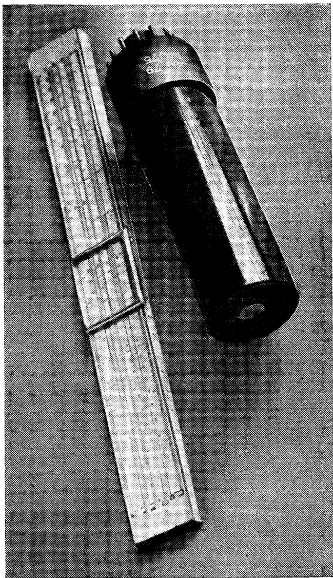
Рис. 55. Внешний вид фотоумножителя ФЭУ-79.
