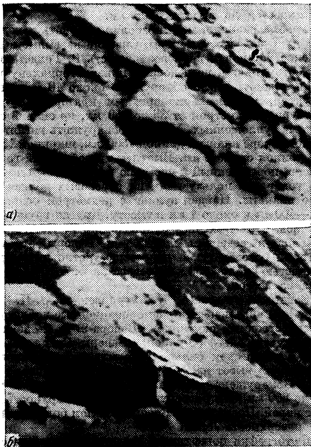
Рис. 24. Части панорам поверхности Венеры, полученные советскими автоматическими станциями «Венера-9» (а) и «Венера-10» (б).
