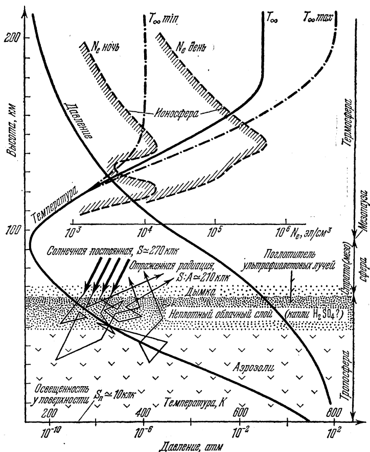
Рис. 22. Модель строения атмосферы Венеры по М. Я. Марову и О. Л. Рябову.
