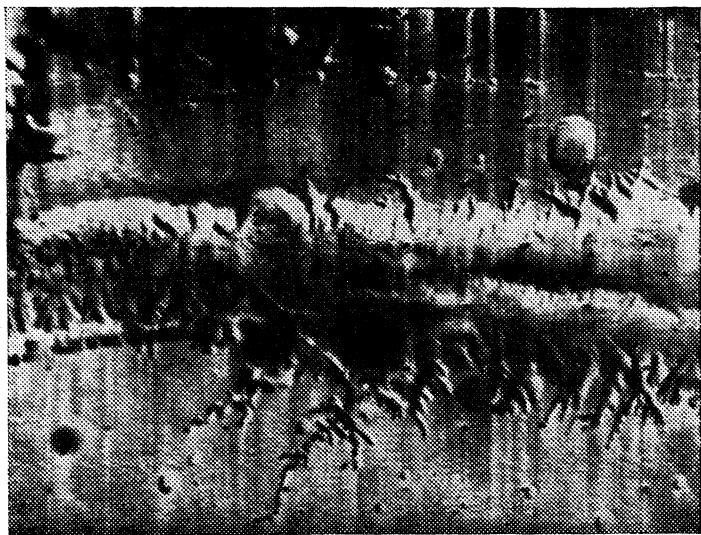
Рис. 27. Разлом Копрат по фотографии «Маринера-9».
