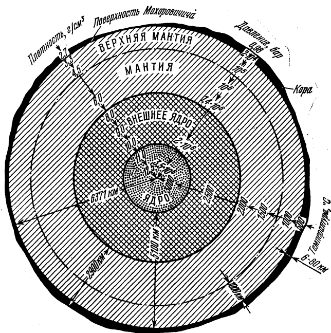
Рис. 42. Внутреннее строение Земли (схема).
