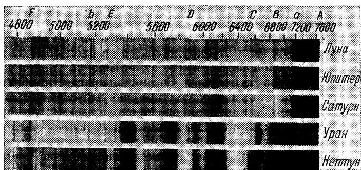
Рис. 12. Спектры Луны и планет-гигантов.
