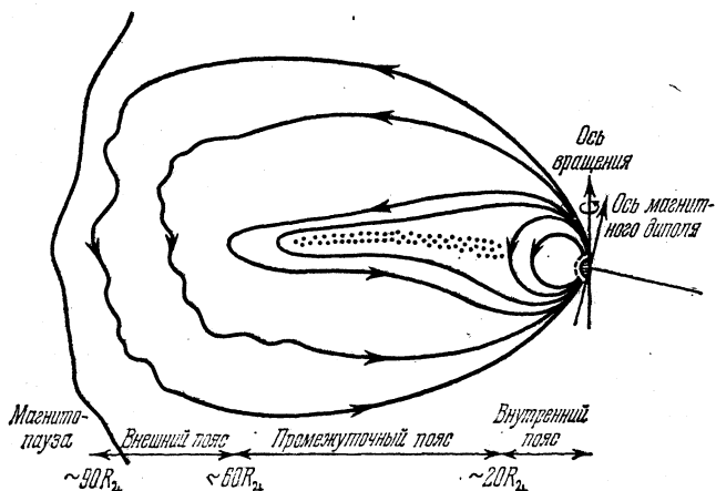
Рис. 33. Строение магнитосферы Юпитера.
