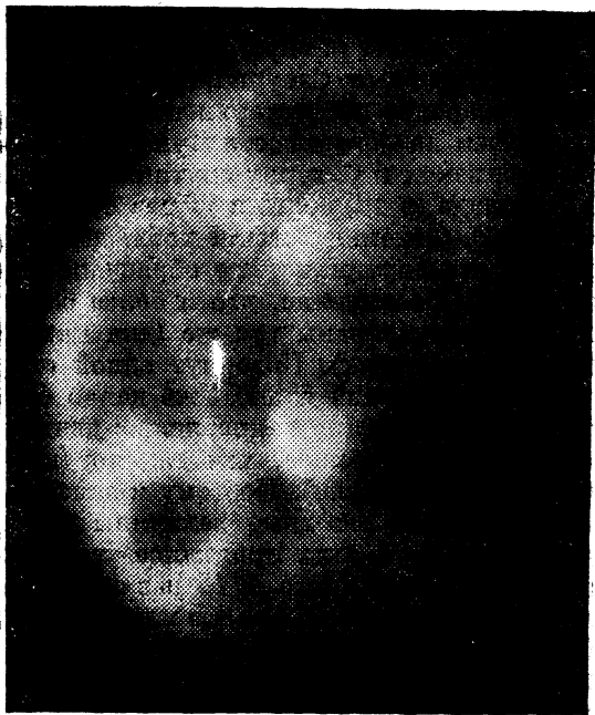
Рис. 37. Фотография Ганимеда, полученная «Пионером-11» в конце 1974 г. Заметно яркое пятно.
