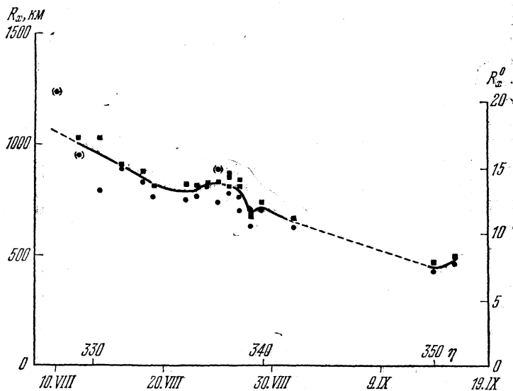
Рис. 48. График таяния полярной шапки Марса в 1956 г. по наблюдениям на обсерватории Волгоградского планетария.
