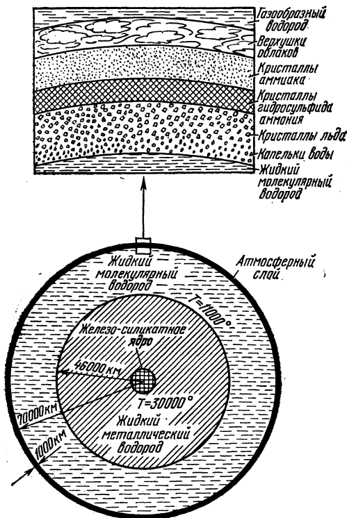
Рис. 43. Внутреннее строение Юпитера (схема).
