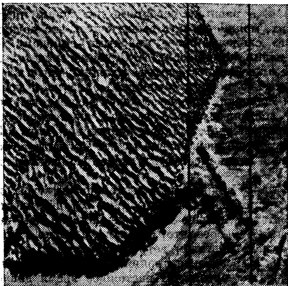
Рис. 28. Дюны на Марсе. Фотография «Маринера-9».
