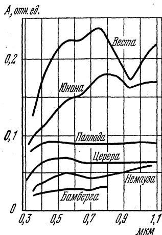
Рис. 40. Отражательная способность астероидов в функции длины волны (по К. Чепмену и Т. Мак-Корду).
