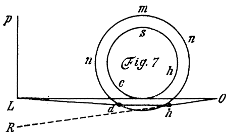
Рис. 4. Схема хода солнечных лучей в атмосфере Венеры (по М. В. Ломоносову). L — точка на краю Солнца, R — ее изображение, представляющееся наблюдателю O .
