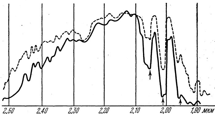
Рис. 11. Регистрограммы спектров Марса (сплошная линия) и Луны (прерывистая), полученные с помощью инфракрасного спектрометра, установленного на 125-сантиметровом рефлекторе Государственного астрономического института им. Штернберга (южная станция в Крыму, В. И. Мороз). Полосы \text{CO}_2 указаны стрелками.
