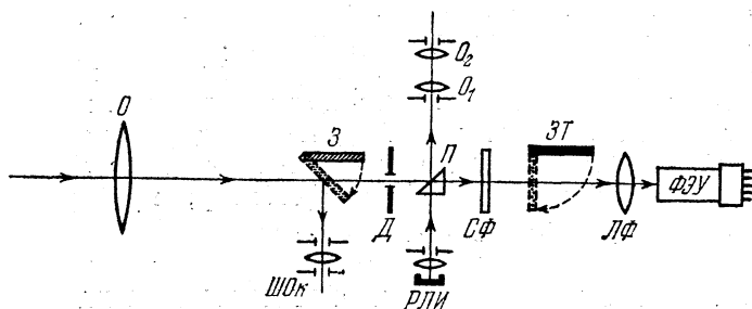
Рис. 54. Принципиальная оптическая схема электрофотометра с ФЭУ. Обозначения см. в тексте.
