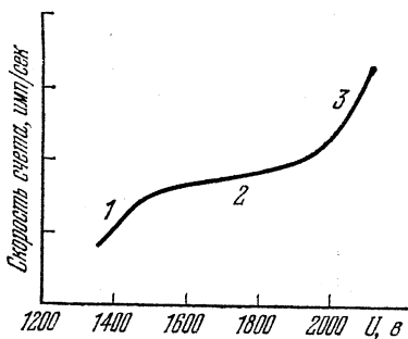
Рис. 58. Примерный вид счётной характеристики фотоумножителя.
