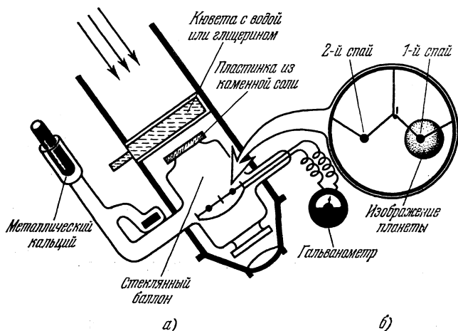
Рис. 8. Схема термоэлемента. Справа — вид поля зрения телескопа с двумя спаями, один из которых проектируется на диск планеты, а другой — на фон неба. Металлический кальций поддерживает вакуум в приборе.
