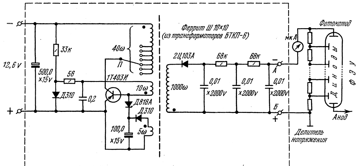
Рис. 57. Схема стабилизированного высоковольтного блока и схема питания фотоумножителя высоким напряжением через простой делитель. Высокое напряжение (до 2300 в) снимается между точками А и Б. Переключатель П служит для его регулировки. Точками обозначены начала обмоток, если все они намотаны в одном направлении.
