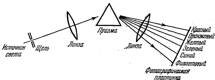
Рис. 10. Схема призмного спектрографа.
