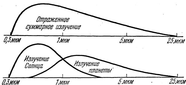
Рис. 9. Составляющие излучения планеты.
