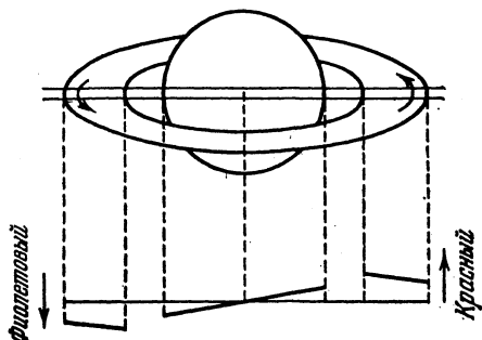
Рис. 13. Схема наклона спектральных линий в спектре Сатурна и его колец.
