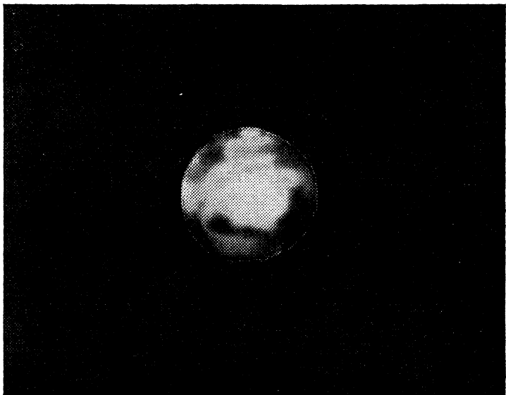
Рис. 25. Фотография Марса, полученная на обсерватории Нью-Мексико (США).
