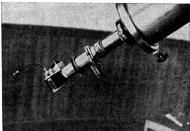
Рис. 52. Окулярная камера типа «Зенит», установленная на 30-сантиметровом рефракторе обсерватории Волгоградского планетария.
