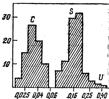
Рис. 41. Распределение астероидов по их альbedo (по Д. Моррисону).
