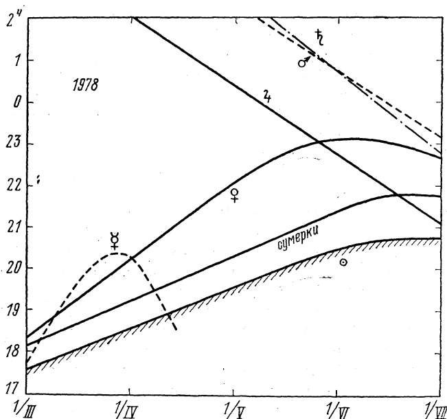
Рис. 45. График вечерней видимости планет в 1978 г.
