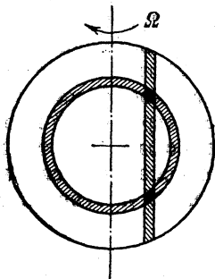
Рис. 17. Метод «запаздывание—Доплер» (схема).
