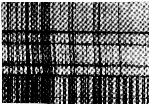
Рис. 14. Спектрограммы Венеры, Сатурна и Луны, полученные с помощью трехпризменного спектрографа. Наклон линий хорошо заметен в спектре Сатурна, но совершенно отсутствует в спектрах Луны и Венеры.
