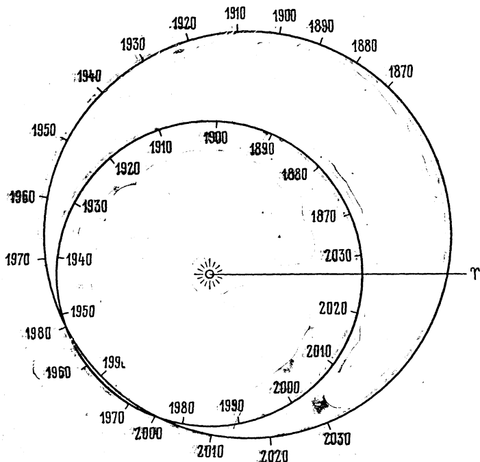
Рис. 35. Орбиты Плутона и Нептуна. Годы указывают положения планет на орбитах.
