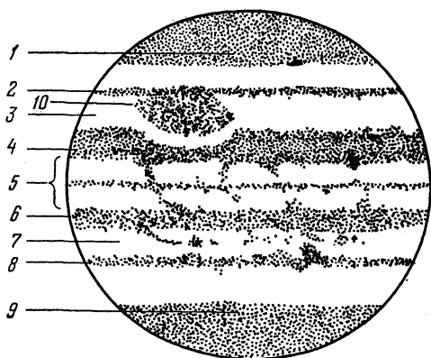
Рис. 49. Схема полос и зон на Юпитере: 1 — S-полярная шапка, 2 — S-умеренная полоса, 3 — S-тропическая зона, 4 — S-тропическая полоса, 5 — экваториальная зона, 6 — N-тропическая полоса, 7 — N-тропическая зона, 8 — N-умеренная полоса, 9 — N-полярная шапка, 10 — Большое Красное пятно.
