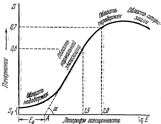
Рис. 7. Характеристическая кривая фотопластинки.
