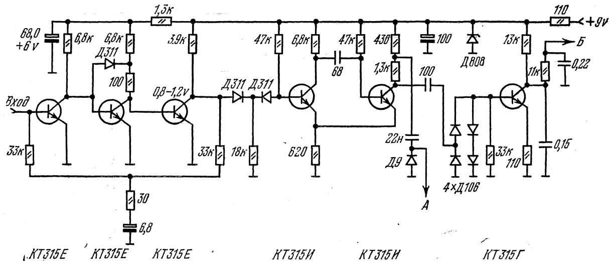
Рис. 56. Схема импульсного транзисторного усилителя для метода счета фотонов.
