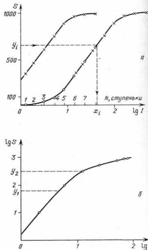
Рис. 29. Построение характеристической кривой: S в линейной шкале (а) и в логарифмической шкале (б)
