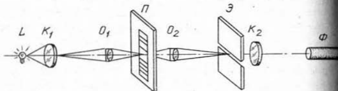
Рис. 18. Оптическая схема микрофотометра
