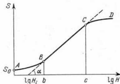
Рис. 9. Характеристическая кривая фотоэмульсии
