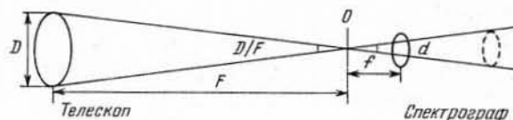
Рис. 15. Согласование телескопа и спектрографа по светосиле
