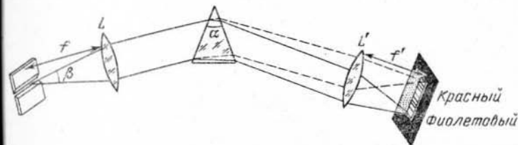
Рис. 11. Схема призмного спектрографа
