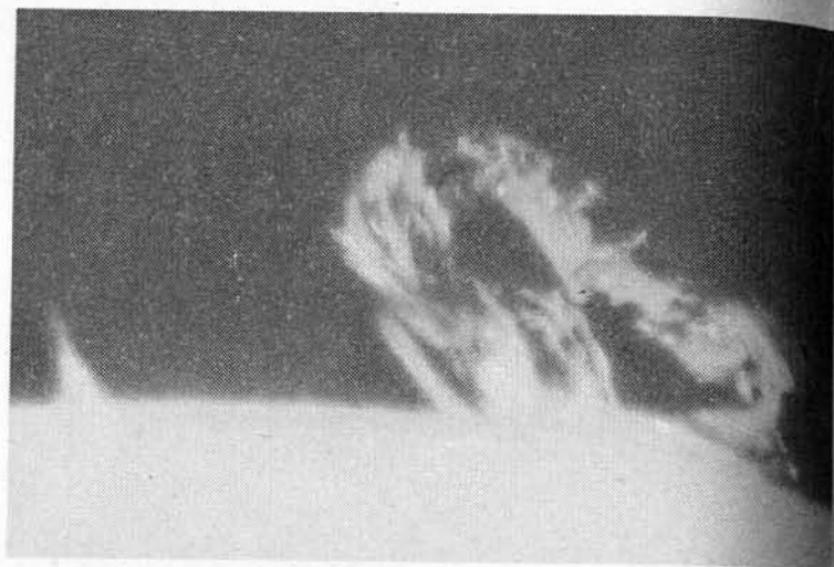
VIIIe. Активный протуберанец
