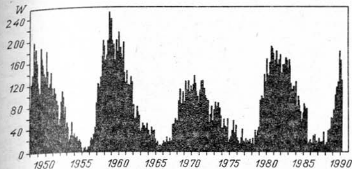
Рис. 23. Изменение относительного числа солнечных пятен (числа Вольфа W ) за четыре 11-летних цикла солнечной активности
