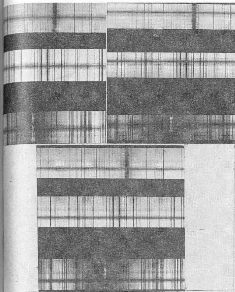
IX. Спектры трех пятен в области Н (верхний спектр на каждой фотографии), в зеленой части спектра ( \lambda=4920 \text{ \AA} ) (спектр в середине) и в области линии К (нижний спектр) (позитив)
