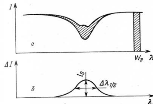
Рис. 32. Характеристики эмиссионного профиля: а — наложение наблюдаемого профиля эмиссионной линии на профиль линии поглощения в соседнем невозмущенном месте Солнца; б — чисто эмиссионный профиль, полученный путем вычитания невозмущенного профиля из наблюдаемого эмиссионного; характеристика этого профиля
