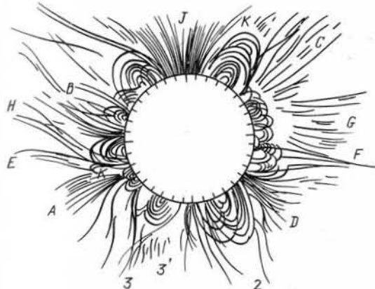
Рис. 34. Типичные структуры, наблюдаемые во внешней короне
