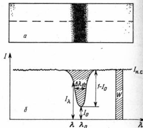
Рис. 31. Основные характеристики профиля спектральной линии поглощения: а — схематическое изображение спектрограммы и направление фотометрического разреза; б — профиль спектральной линии поглощения и его характеристики
