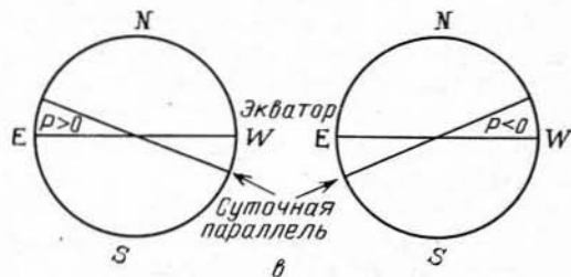
Рис. 20. Проведение суточной параллели по пятну (а), по касательной к диску (б); проведение экватора в зависимости от знака P (в)
