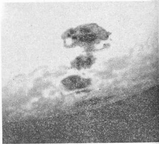
III. Слева — фотосфера Солнца недалеко от восточного края диска. Видна выходящая из-за края большая группа пятен, окруженная яркими факелами. Зернистая структура окружающей фотосферы — грануляция. Справа — хромосфера Солнца. Видна большая группа пятен, сфотографированная в линии H_{\alpha} . В центре — самая яркая часть фотосферы — более темные небольшие волокна.
