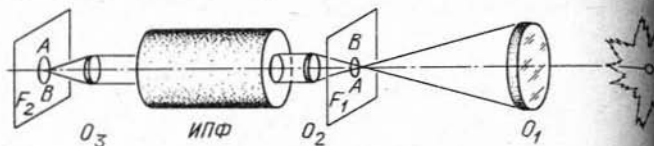
Рис. 17. Схема установки интерференционно-поляризационного фильтра (ИПФ) на телескопе
