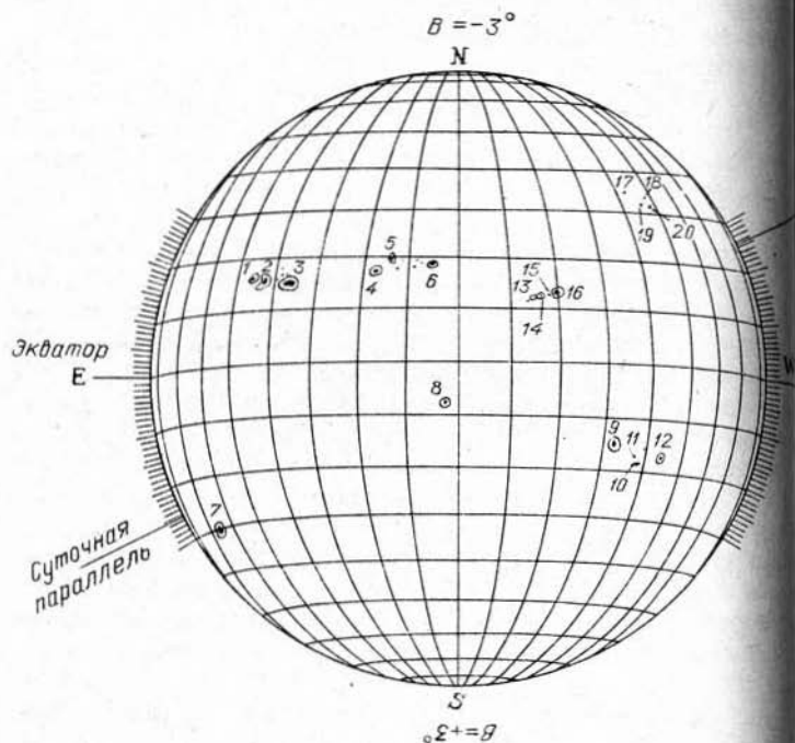
Рис. 21. Зарисовка Солнца, нанесенная на координатную сетку
