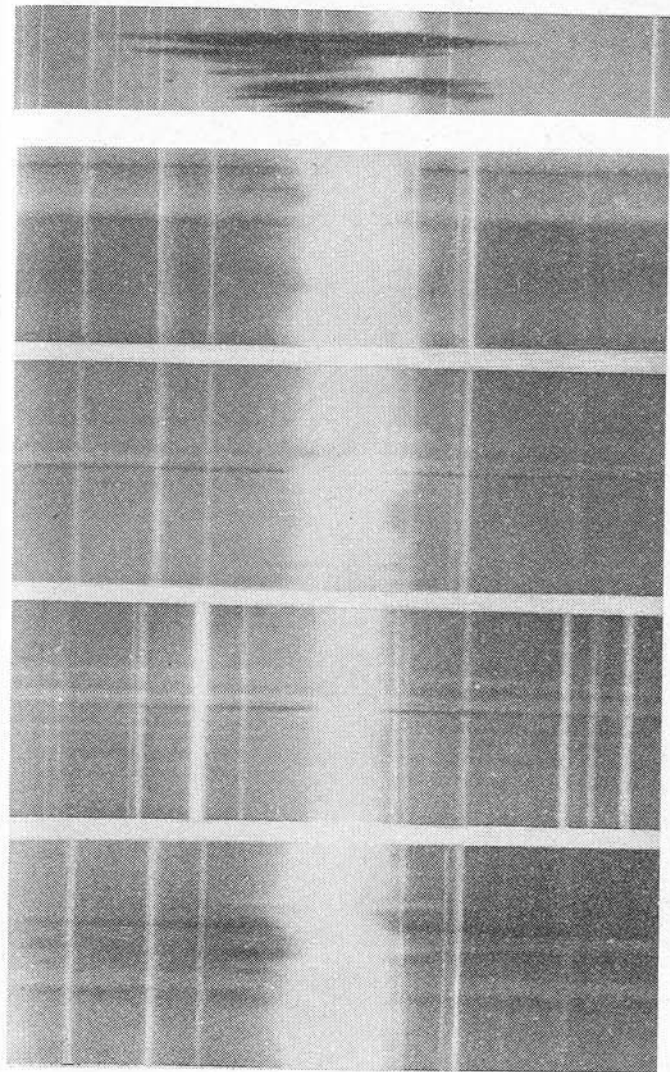
XII. Вверху — спектр протуберанца в области линии H_\alpha (негатив). Более слабые линии, непрерывный спектр и линии поглощения, принадлежат рассеянному свету неба. Темная (на самом деле яркая) эмиссия — излучение протуберанца в линии H_\alpha , смещенная по спектру в синюю сторону от линии поглощения H_\alpha из-за движения с большой скоростью от Солнца к наблюдателю (эффект Доплера). Внизу — усы в линиях водорода H_\alpha (спектры 1-й, 2-й и 4-й сверху) и H_\beta (3-й спектр) (негатив)
