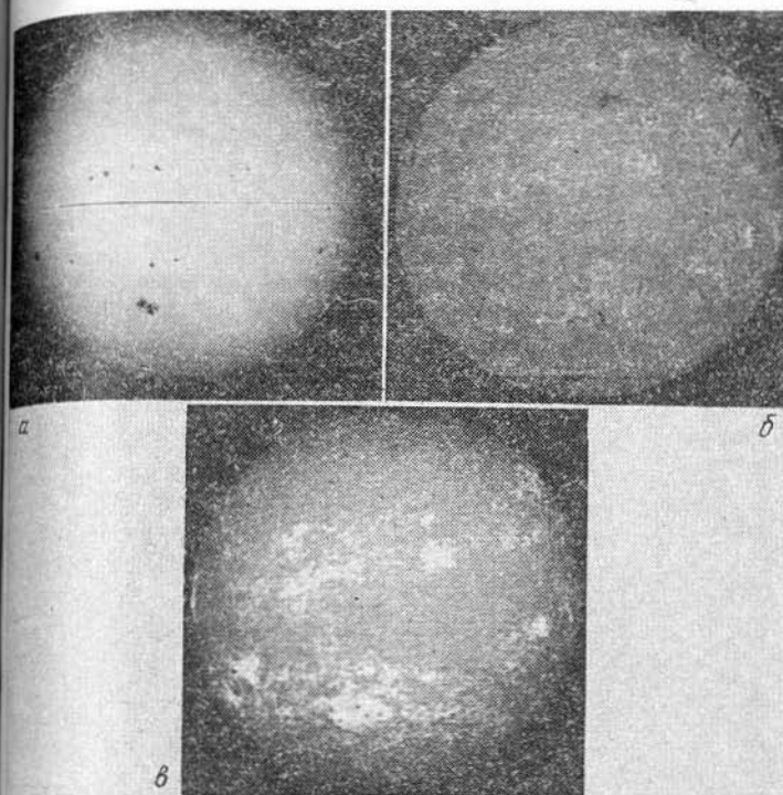
1. Вид диска Солнца в белом свете (а), в линии водорода H_\alpha (б), в линии К ионизованного кальция (в)
