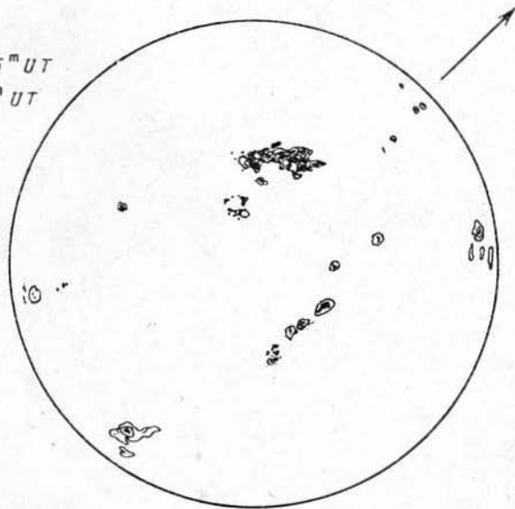
XIV. Зарисовка Солнца 16 июня 1989 г. Стрелка показывает направление суточной параллели
