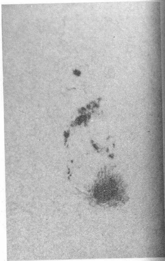
Иа. Група пятен в белом свете
