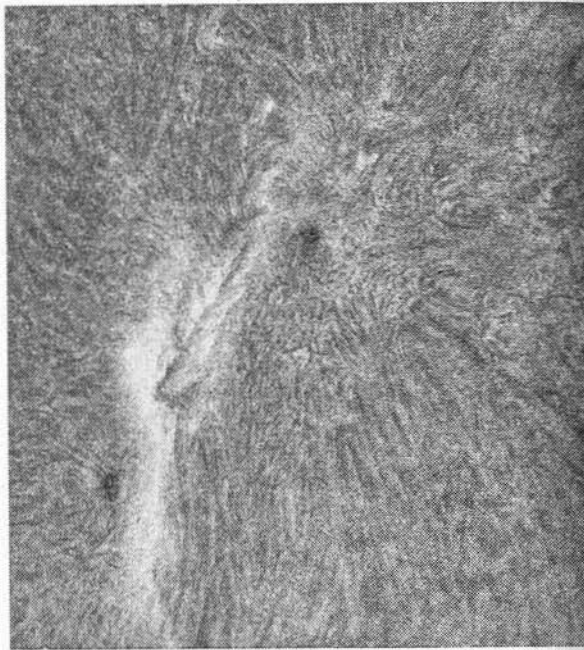
III. Слева — фотосфера Солнца недалеко от восточного края диска. Видна выходящая из-за края большая группа пятен, окруженная яркими факелами. Зернистая структура окружающей фотосферы — грануляция. Справа — хромосфера Солнца. Видна большая группа пятен, сфотографированная в линии H_{\alpha} . В центре — самая яркая часть фотосферы — более темные небольшие волокна.
