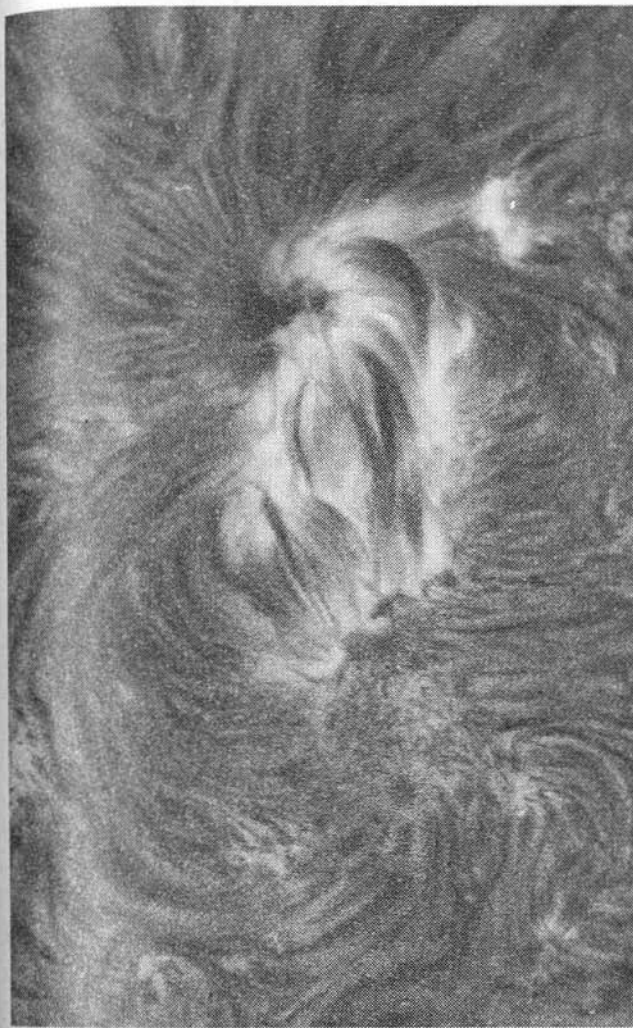
Иб. Та же группа в линии H_{\alpha}
