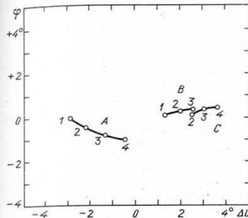
Рис. 26. Собственные движения трех пятен A, B, C. Цифры означают дни наблюдений
