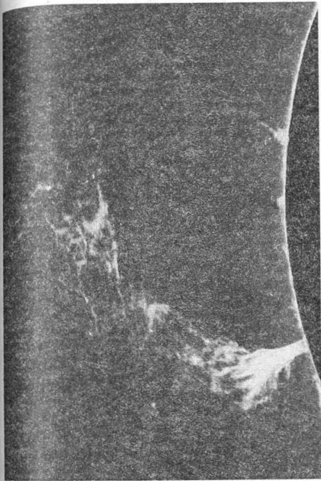
III. Слева — фотосфера Солнца недалеко от восточного края диска. Видна выходящая из-за края большая группа пятен, окруженная яркими факелами. Зернистая структура окружающей фотосферы — грануляция. Справа — хромосфера Солнца. Видна большая группа пятен, сфотографированная в линии H_{\alpha} . В центре — самая яркая часть фотосферы — более темные небольшие волокна.
