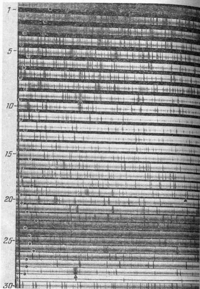
Ха. Левая часть спектра Солнца, полученного на спектрографе с решеткой-эшеле (позитив)
