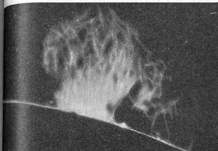
VIIIa. Спокойный протуберанец (все снимки протуберанцев в линии H_2 )
