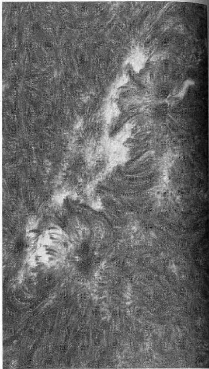
Vа. Снимок хромосферы в линии H_2 .
