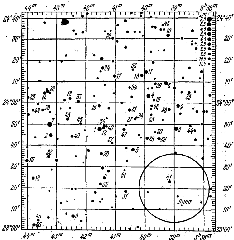
Рис. 50. Вид Плеяд в телескоп (кружком обозначены размеры лунного диска): 1 — Альциона, 2 — Атлас, 3 — Электра, 4 — Майя, 5 — Меропя, 6 — Тайгета, 7 — Плейона, 9 — Целена, 11 — Астеропа.
