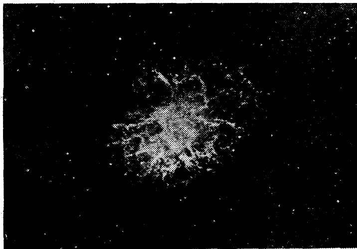
Рис. 54. Крабовидная туманность.
