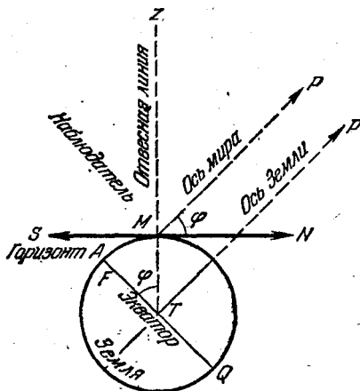
Рис. 25. Теорема о высоте полюса кого-нибудь географического мира.
