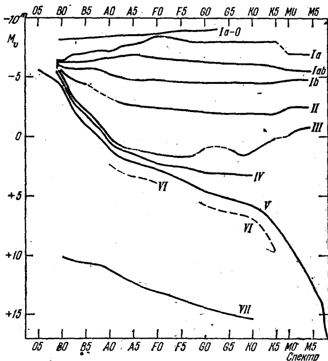
Рис. 3. Диаграмма Герцшпрунга — Рассела. Последовательности: Ia-0 — ярчайших сверхгигантов, Ia — ярких сверхгигантов, Iab — средних сверхгигантов, Ib — слабых сверхгигантов, II — ярких гигантов, III — слабых гигантов, IV — субгигантов, V — главная последовательность, VI — субкарликов, VII — белых карликов.
