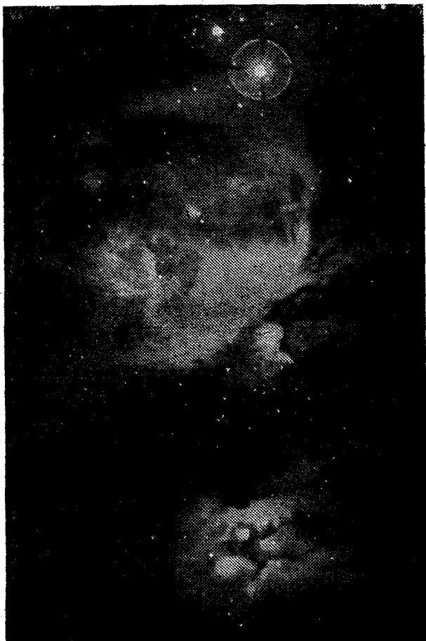
Рис. 49. Туманность Ориона.
