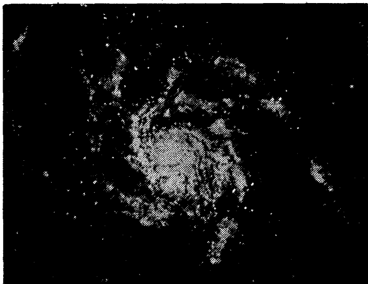
Рис. 33. Галактика М 101.
