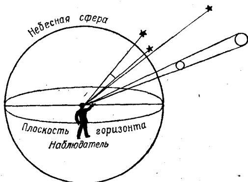
Рис. 19. Небесная сфера.
