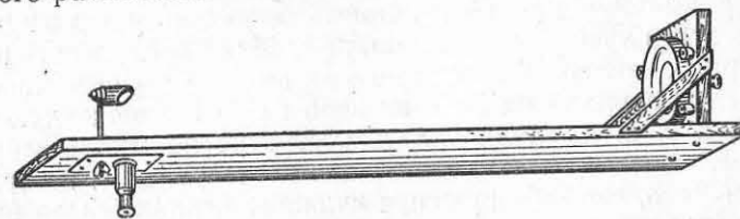
Рис. 6. «Чикинская доска» для предварительной монтировки. Описанное в тексте устройство окулярной части доски несколько упрощено по сравнению с показанным на рисунке
