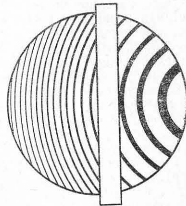
Рис. 5. Вид интерференционных полос в случае выпуклости испытуемого стекла (предполагается, что на него наложено в точности плоское пробное стекло). С правой стороны полосы шире и сильнее искривлены, что указывает на более тесное соприкосновение стекол. Приложенная линейка позволяет определить кривизну стекла (в данном случае выпуклость составляет около трех полос)
