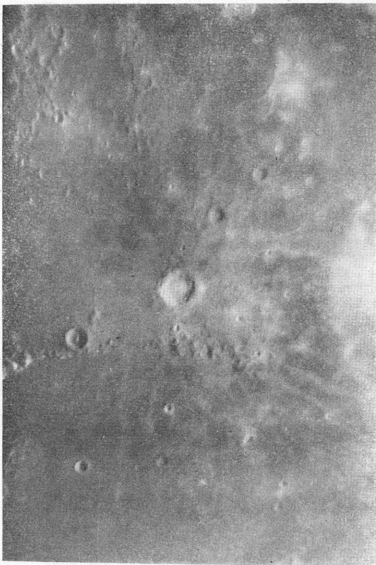
Рис. 8. Фотография части лунного диска близ кратера Коперник, полученная около последней четверти в касегреновском фокусе 320-миллиметрового рефлектора, построенного А. С. Фоминым.
