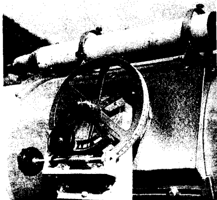
Механизм поворота относительно оси склонений
