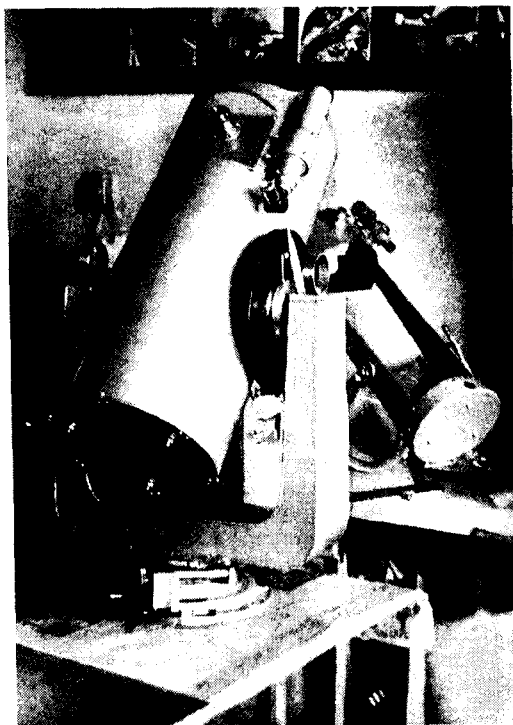
Общий вид самодельного менискового теле- скопа
