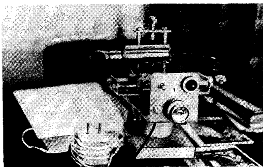
Теновый прибор, в котором щель, нож и нить располагаются вертикально
