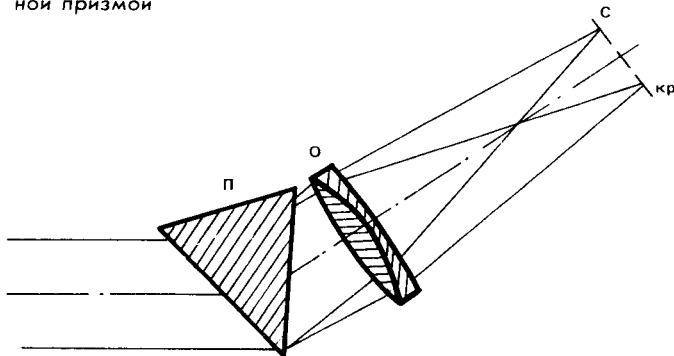
Схема астрографа с объективной призмой
