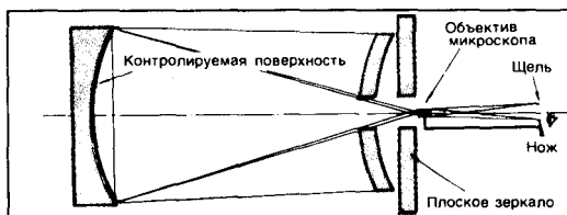
Схема контроля выпуклой поверхности мениска и системы «мениск — главное зеркало»
