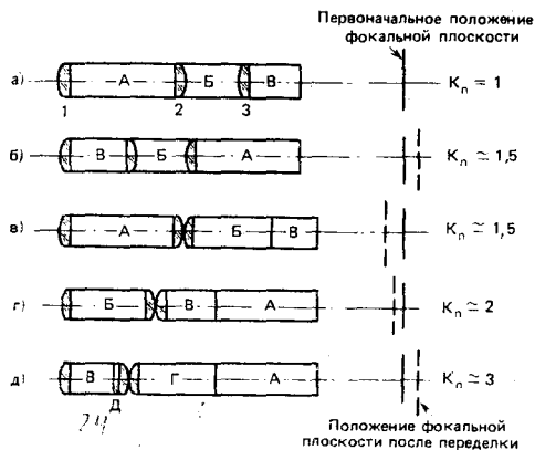
Оптическая схема зрительной трубы «Турист»
