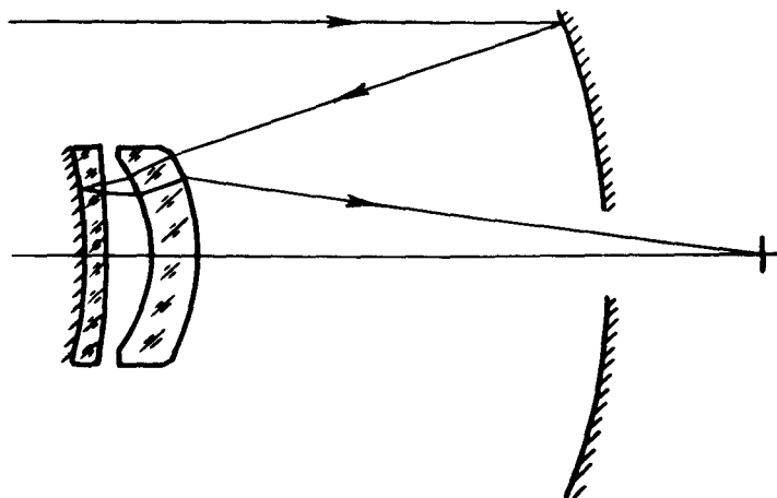
Оптическая система телескопа с менисковым корректором
