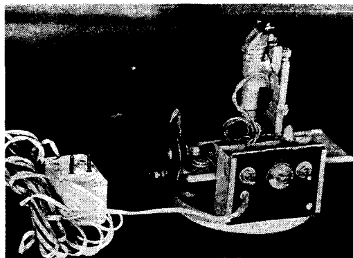
Теновый прибор, выполненный на основе фотоаппарата «Фотокор»
