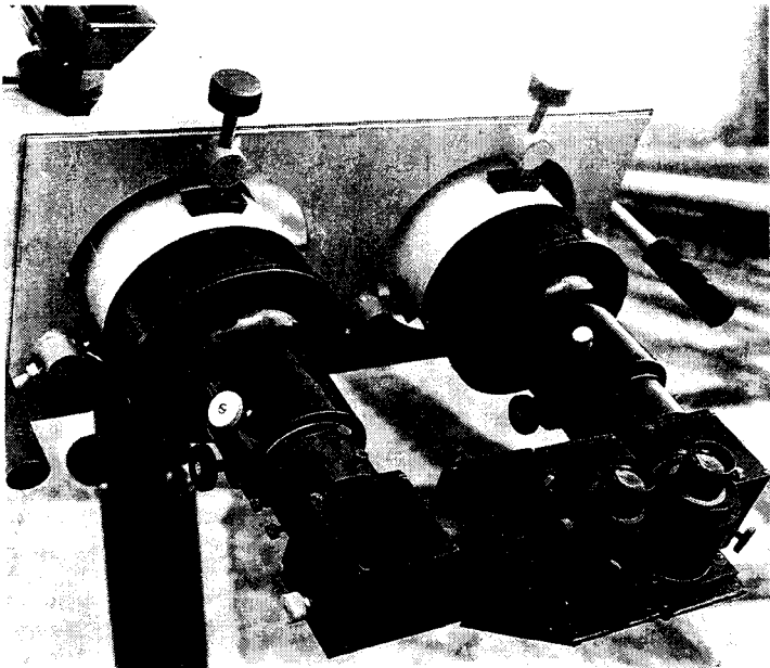
Окулярный узел
