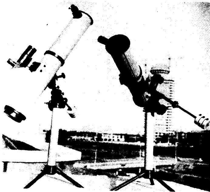
Переносные 120- и 125-миллиметровые телескопы системы Ньютона, изготовленные М. Морозовым, Д. Тепловым и К. Шайхатдиновым (Красноярский краевой Дворец пионеров и школьников)
