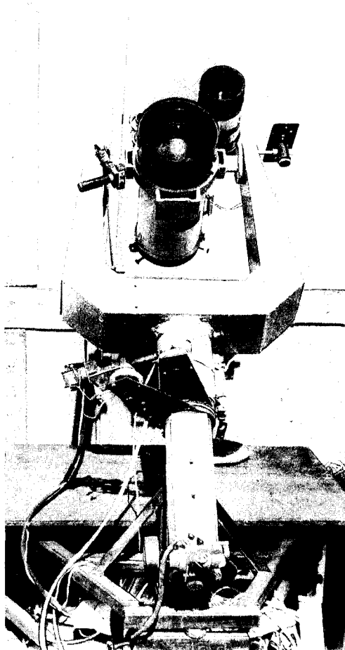
Астрограф с объективом «Уран-12». Ниже вилки видны два рычага с механизмом тонких движений по прямому восхождению
