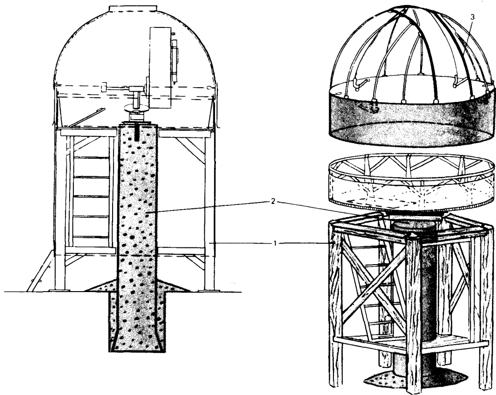
Схема купола. 1 — каркас башни, 2 — труба-фундамент телескопа
