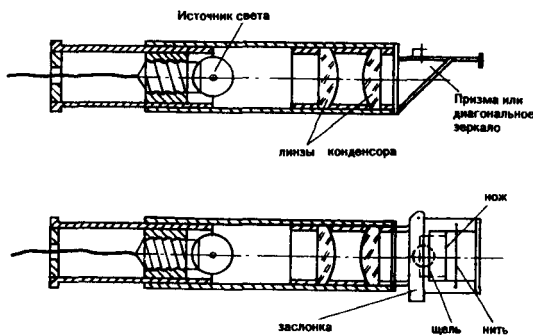
Схема комбинированной головки теневого прибора
