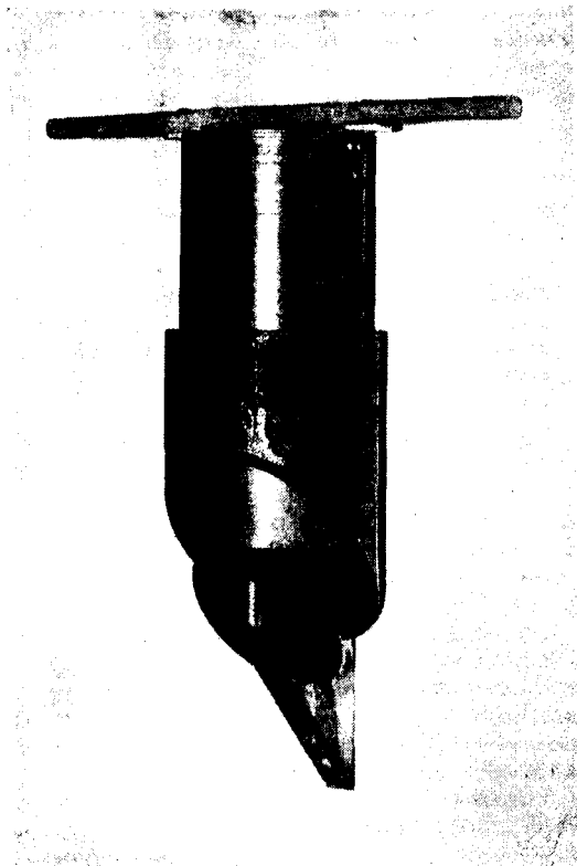
Приспособление для вырезания заготовки эллиптического очертания
