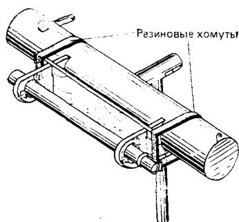
Искатель на телескопе «Алькор»
