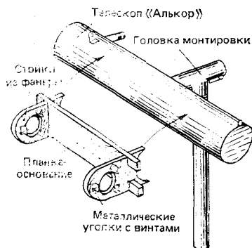
Устройство для крепления искателя
