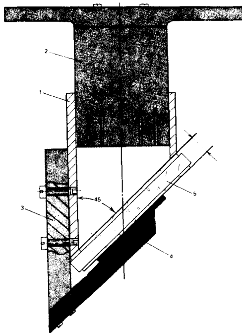
Схема приспособления для вырезания заготовок эллиг.ической формы: 1 — корпус, 2 — трубчатое сверло, 3 — кронштейн, 4 — кронштейн с поддерживающей лапкой, 5 — заготовка с подклеечными стеклами
