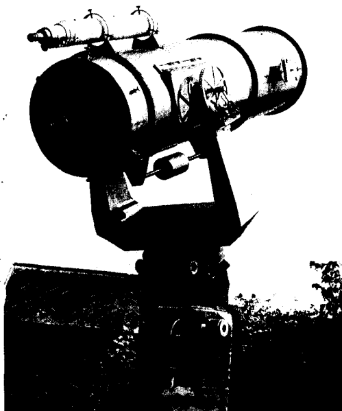
400-миллиметровый рефлектор системы Ньютона—Кассегрена
