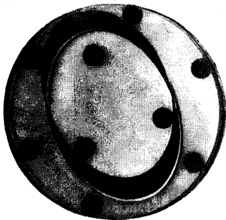
Заготовка зеркала и вспомогательное стекло, наклеенные на основание-план
