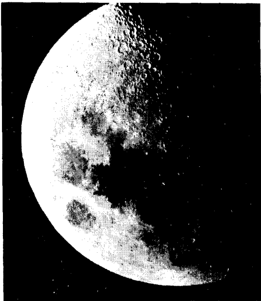
Снимки Луны, полученные на 180-миллиметровом телескопе
