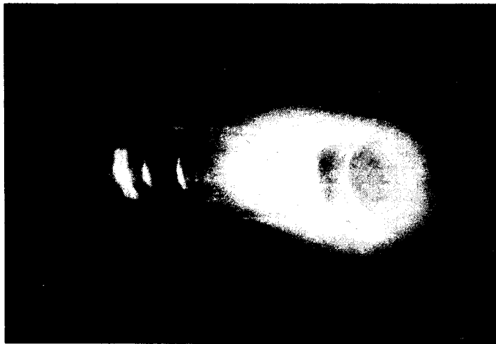
Спектр хромосферы и короны Солнца. Хорошо заметны линии кальция, водорода, магния. (Слева — синий конец спектра). Пленка «Kodak-64», увеличение при печати — 10 x
