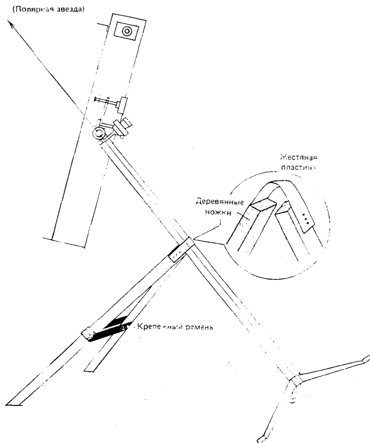
Простейшая экваториальная монтажка для «Алькора»
