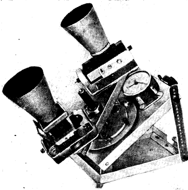
Общий вид астрографа
