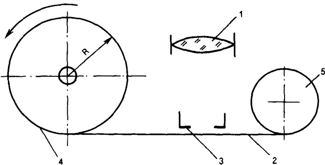
Схема работы астрографа: 1 — объектив, 2 — фотопленка, 3 — кадрирующая рамка, 4 — барабан, 5 — кассета
