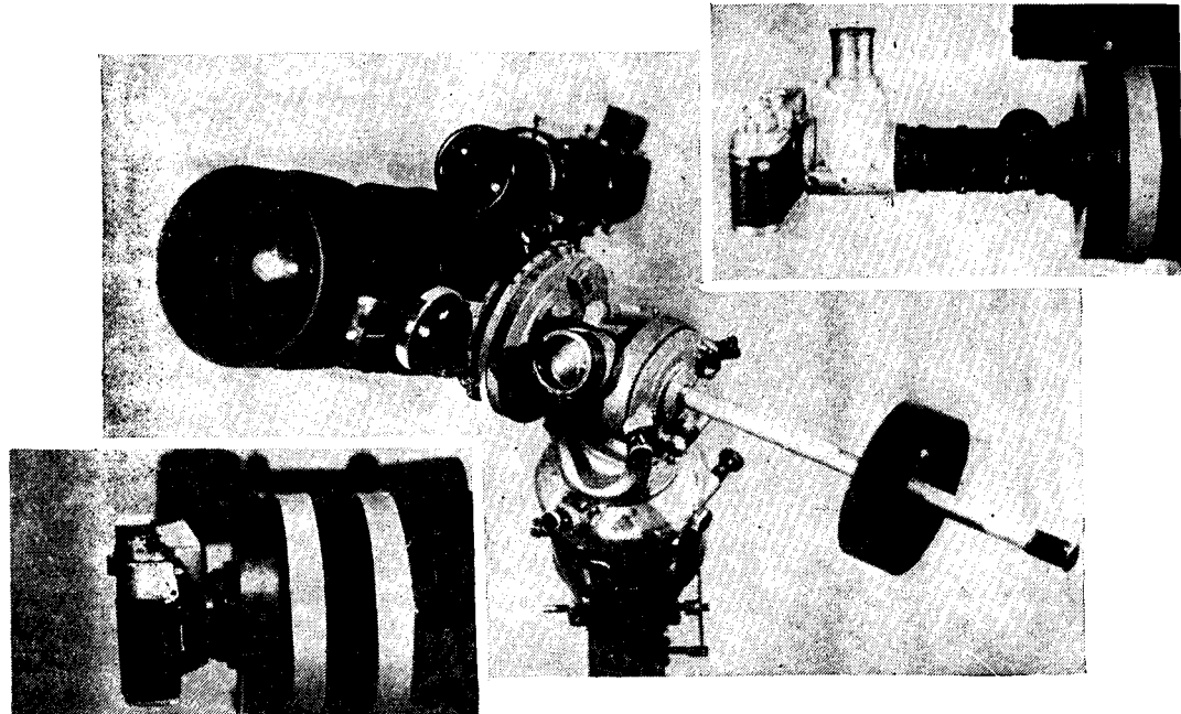
Самодельный телескоп, основой которого стал фотообъектив «МТО-1000», монтировка немецкого типа. Вверху: окулярная камера в эквивалентном фокусе F=5000 мм. Внизу: фотоаппарат «Зенит» в штатном фокусе (1100 мм)
