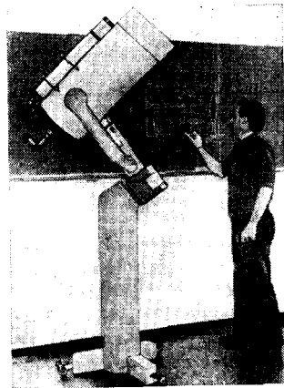
320-мм телескоп системы Шмидта — Кассегрена, построенный Л. Нийборгом (Нидерланды)
