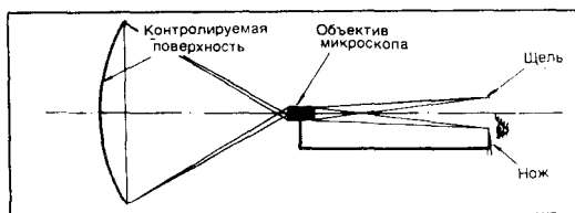
Схема контроля светосильных зеркал
