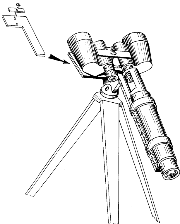
Телескоп из бинокля. Второй монокуляр бинокля используется в качестве искателя
