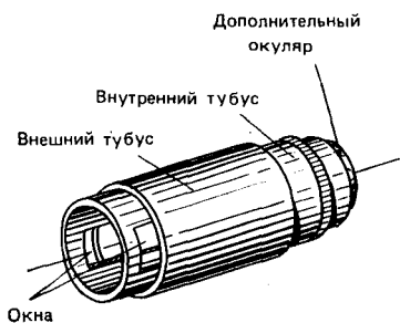
Крепление дополнительного окуляра, обеспечивающее плавное изменение увеличения инструмента
