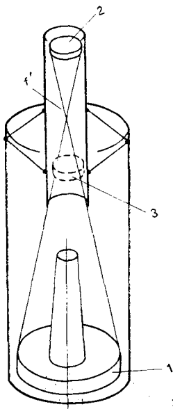
2,08-метровый телескоп обсерватории Макдональд
