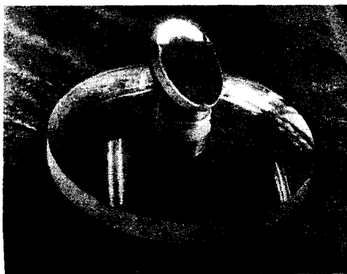
Мениск и вспомогательное зеркало с опра- вой и юстировочным устройством
