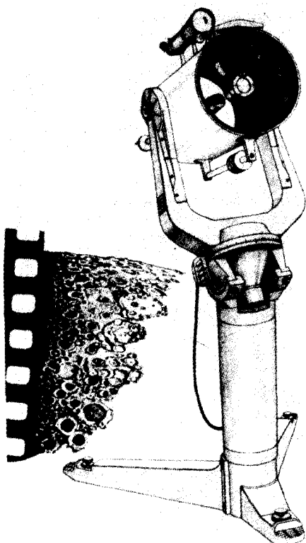
Общий вид 200-миллиметрового телескопа системы Кассегрена с кольцевой опорой
