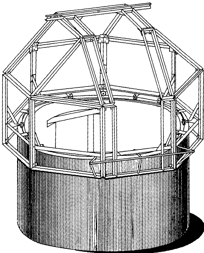
Многогранный купол с восьмиугольным основанием
