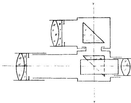
Схема фотометра
