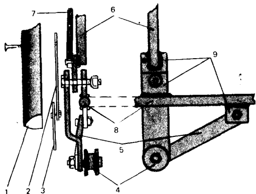
Схема обшивки купола и роликовой опоры. 1 — желоб, 2 — сегмент обшивки, 3 — цилиндрическая часть купола, 4 — ролик, 5 — укосина стойки ролика, 6 — дуга купола, 7 — фанера, 8 — окружность каркаса купола, 9 — крепление пластины
