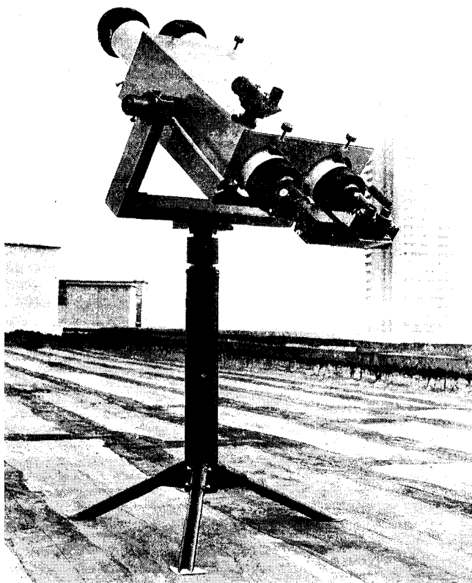
Общий вид 150-миллиметрового бинокляра
