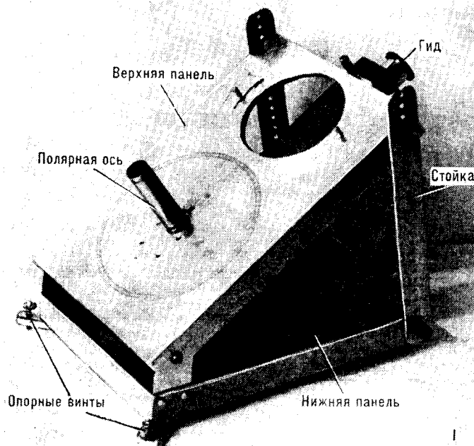
Основные узлы астрографа: 1 — экваториальная монтировка; 2 — зубчатое колесо с вмонтированными в прямоугольные вырезы шариковыми подшипниками; 3 — часовой механизм астрографа на экваториальной монтировке
