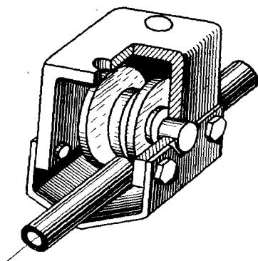
Ограничитель раздвижной створки купола
