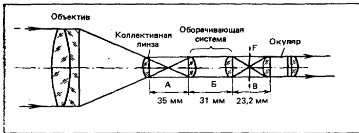
Оптическая схема зрительной трубы «Турист»
