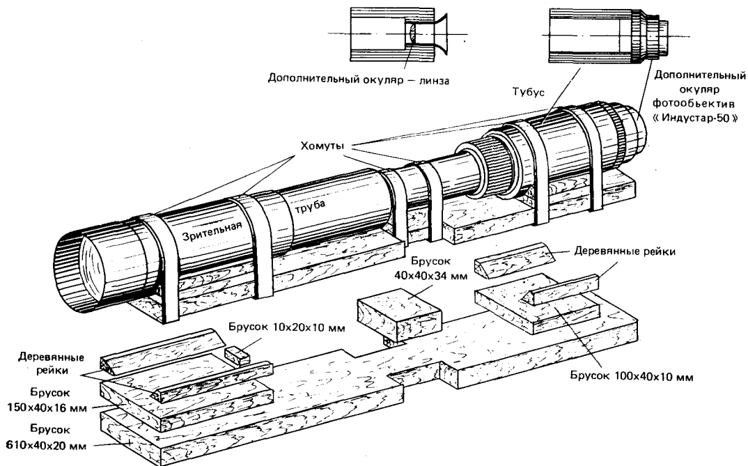
Схема крепления зрительной трубы с дополнительным окуляром на деревянной подставке
