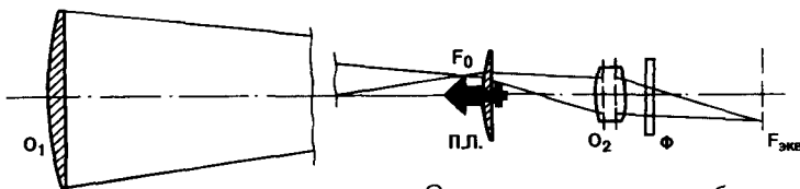
Оптическая схема протуберанц-телескопа
