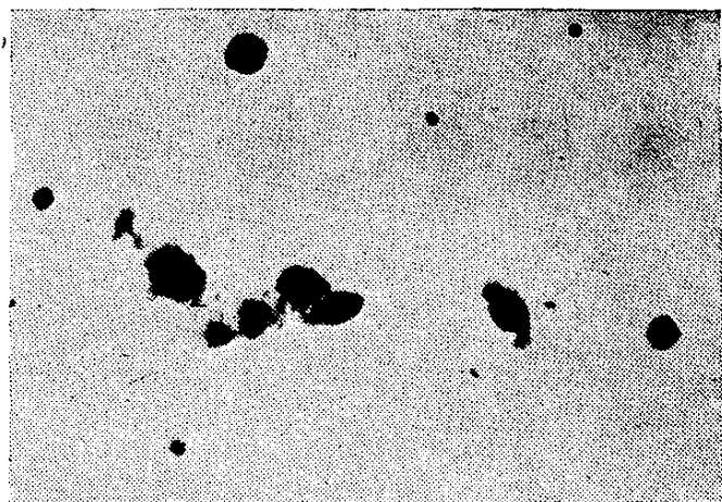
Рис. 90. Цепочка взаимодействующих галактик VV 165.
