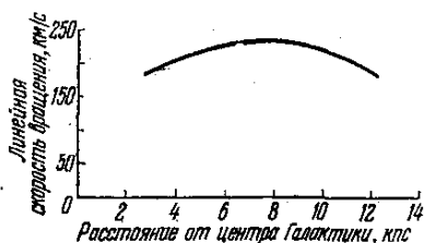
Рис. 10. Закон изменения линейной скорости вращения в Галактике.
