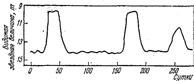
Рис. 6. Изменение блеска U Близнецов.
