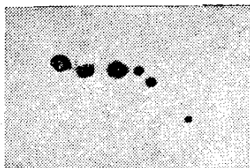
Рис. 91. Цепочка взаимодействующих галактик VV 172.
