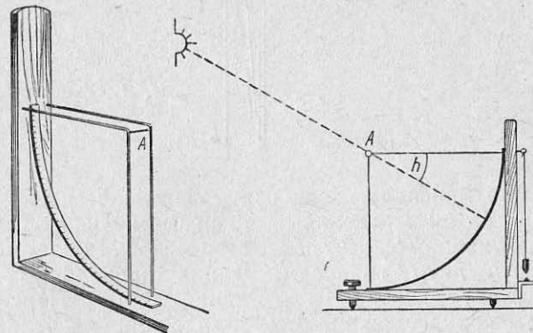
Рис. 6. Квадрант-высотомер
