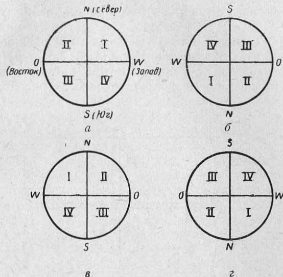
Рис. 19. Расположение стран света при наблюдении Солнца:
