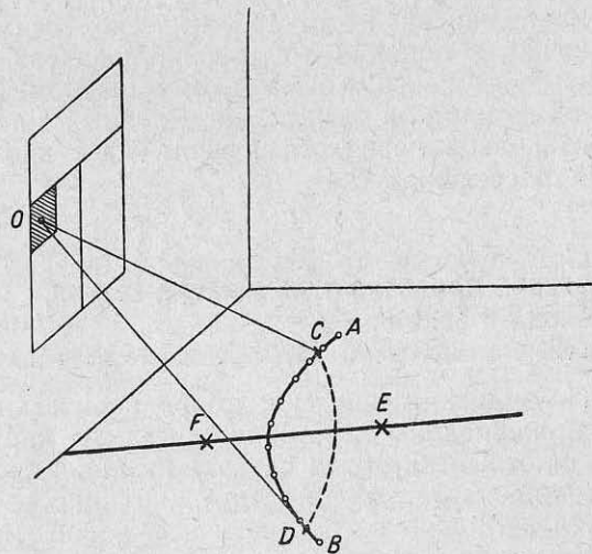
Рис. 14. Определение направления меридиана в классной комнате
