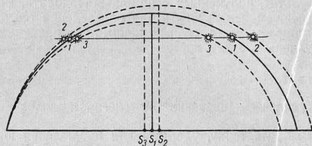
Рис. 12. Дневной путь Солнца по небосводу:
