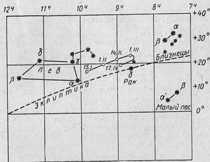
Рис. 15. Видимый путь Марса в январе — апреле 1963 г.
