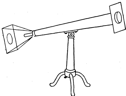
Рис. 40. Проектирование Солнца на экран.
