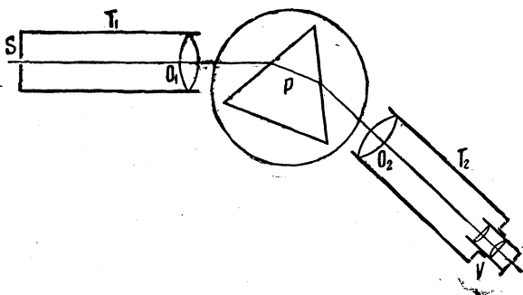
Рис. 1. Схема спектроскопа.
