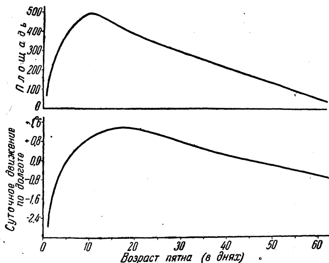
Рис. 17. График развития головного пятна группы. Вверху — изменение площади пятна, внизу — собственное движение (смещение пятна по долготе относительно его среднего положения).
