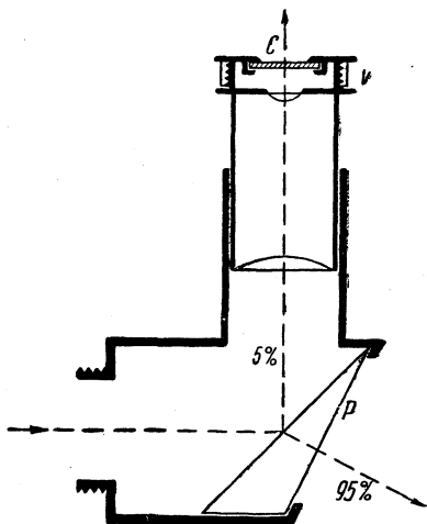
Рис. 38. Схема гелиоскопического окуляра Гершеля.
