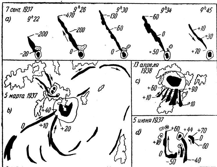
Рис. 27. Волокна, окружающие солнечные пятна.
