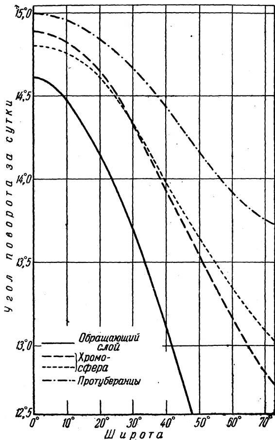
Рис. 7. График, показывающий изменение скорости вращения Солнца с широтой (угол поворота в градусах за сутки, полученный спектроскопическим путём), для разных слоев солнечной атмосферы.
