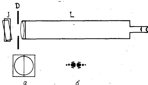
Рис. 3.5. Принцип работы звездного интерферометра Данжона. a — компенсатор Жамэна ( J ), состоящий из двух одинаковых плоскопараллельных пластинок, которые помещаются перед объективом, б — диафрагма ( D ) ограничивает отверстие и изменяет вид изображения. (Рисунок заимствован из Ann. Obs. Strasbourg .)
