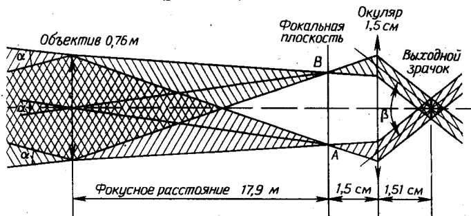
Рис. 2.1. Телескоп-рефрактор. Схема построения изображения. Увеличение. Объектив строит изображение AB компонентов двойной звезды в фокальной плоскости. В окуляр изображение AB видно под углом \beta , большим, чем угол \alpha . Для наглядности схема дана в произвольном масштабе. Приведены реальные размеры большого рефрактора в Ницце. Для двойной звезды Кастор \alpha = 2,20'' , \beta = 44' , AB = 0,192 мм, увеличение \beta/\alpha = 1200 . Диаметр выходного зрачка 0,63 мм.
