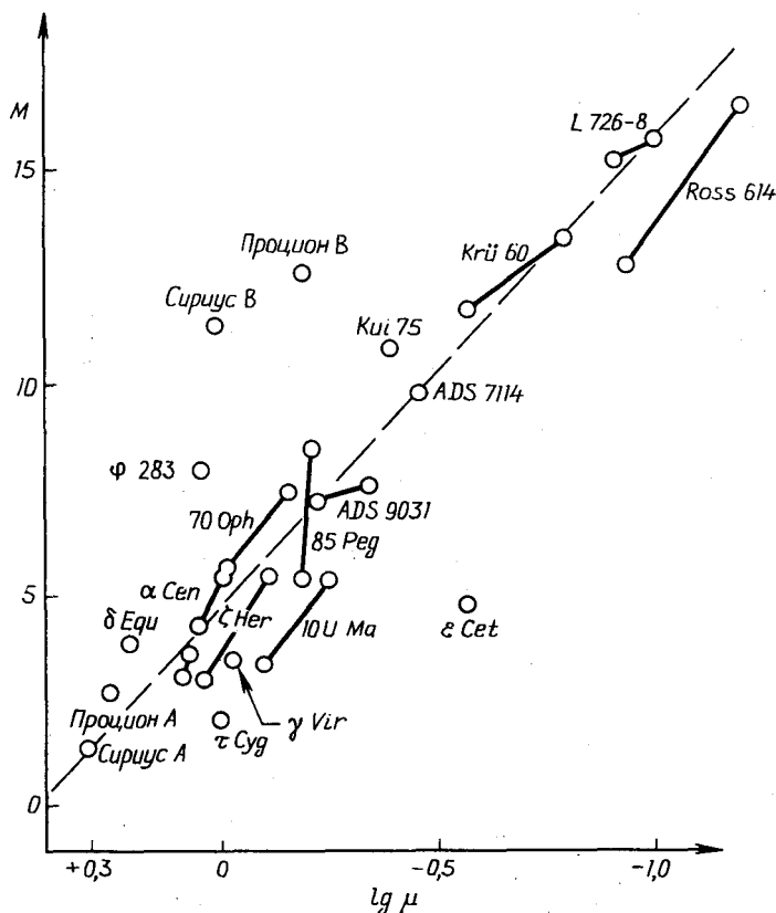
Рис. 6.14. Число используемых звезд ограничено, чтобы не загружать рисунок. Компоненты пары соединены отрезками прямых. Пунктирная линия приведена в соответствии с соотношением Бэза — Романи. По оси абсцисс отложен логарифм массы в долях M_{\odot} .
