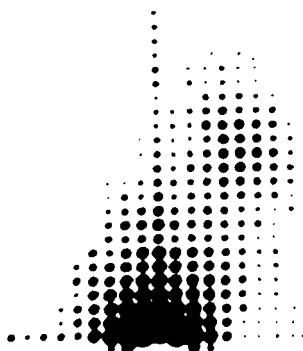
Рис. 3.15. Изображение \beta Северной Короны, полученное методом автокорреляционного анализа. Север внизу. Позиционный угол спутника 150^\circ , расстояние от главной звезды 0,30'' . (Фото Лябери, обсерватория Маунт-Паломар.)
