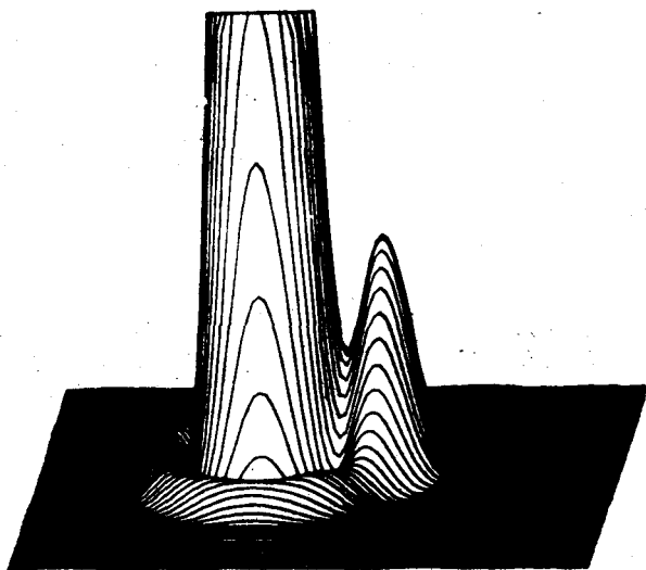
Рис. 2.7. Изофоты двойной звезды с неодинаковыми компонентами. (Фотография С. D. C. A.)
