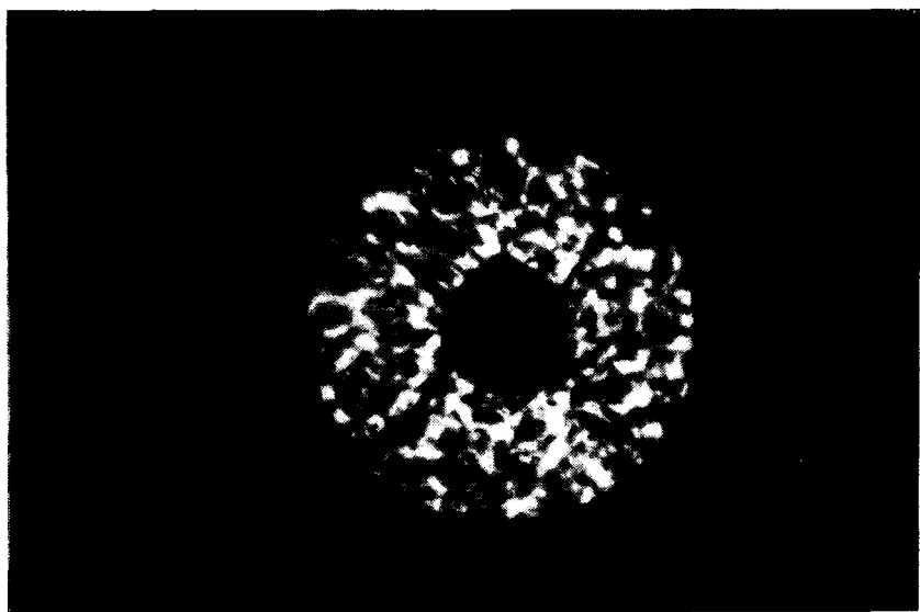
Рис. 4.9. Фотография блуждающих теней. Тени сфотографированы на рефлекторе с апертурой 152 см обсерватории От-Прованс Мартином и Борньино (Университет в Ницце). Экспозиция 1/1000 с, увеличение яркости в 80 000 раз, пленка Tri X. В отсутствие турбулентности поверхность зеркала выглядела бы равномерно освещенной. Видна тень от вторичного зеркала (система Кассегрена) и силуэты растяжек, удерживающих вторичное зеркало.
