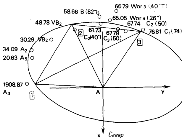
Рис. 6.6. Иллюстрация метода Тилля—Иннеса—ван ден Боса. Приведены данные для двойной звезды ADS 1227 = A 1913. Нанесены результаты наблюдений, а также сокращенное имя наблюдателя, число ночей, отверстие инструмента в дюймах (") или в сантиметрах. Видимый эллипс проведен по трем средним местам.
