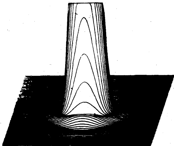
Рис. 2.5. Изофоты неразрешенной двойной звезды, блеск компонентов которой одинаков. (Фотография С.Д.С.А.) Можно заметить две симметричные пучности света в первом кольце.
