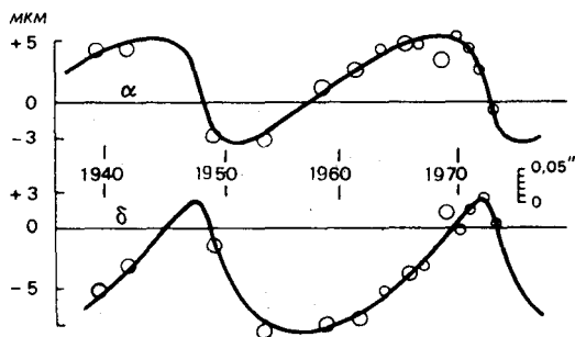
Рис. 6.12. Возмущенная траектория звезды, имеющей невидимый спутник. (Lippincott S. L. Astron J., с разрешения автора и издателя.) Звезда BD + 67°552. Движения по прямому восхождению и склонению отклоняются от прямолинейной траектории, что связано с присутствием невидимого спутника. Эти отклонения достигают 5 мкм в фокусе рефрактора обсерватории Спрул. Размеры кружков представляют вероятные ошибки наблюдений. Диаметр измеряемого фотографического изображения составляет около сотни микрометров. P = 23,0 года, T = 1949,0 , e = 0,73 .
