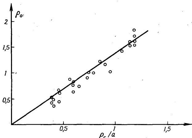
Рис. 6.8. Измерение большой оси ADS 10786 = AC 7. По оси абсцисс отложены вычисленные величины \rho_c/a , по оси ординат — измеренные разделения \rho_0 . Точки ложатся около прямой, наклон которой определяет большую полуось. Нанесены лишь некоторые наблюдения.
