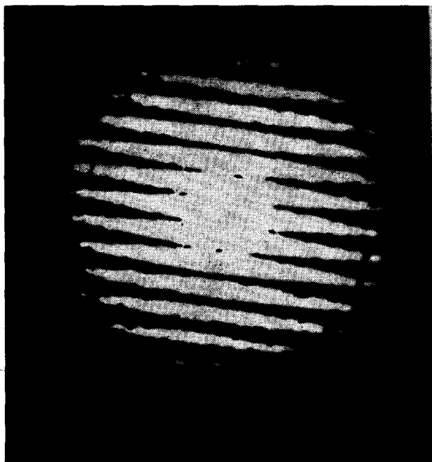
Рис. 3.14. Интерференционная картина изображения \chi Большой Медведицы. Получена сложением 50 фотографических изображений, снятых на 4-метровом рефлекторе обсерватории Китт-Пик. Угловое разделение компонентов составляет 0,272'' . (Фото Мак-Алистера, опубликованное в Sky and Telescope ; с разрешения автора и издателя.)
