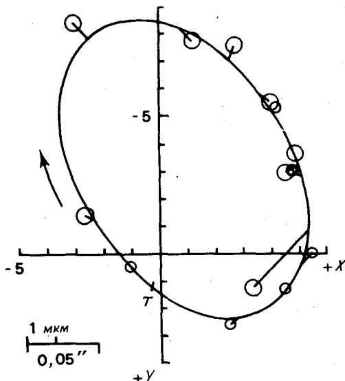
Рис. 6.13. Орбита фотоцентра звезды BD + 67°552. ( Lippincott S. L. Astron. J. , с разрешения автора и издателя.) Эта орбита построена на основе анализа траекторий, изображенных на рис. 6.12. Размер траектории не превышает 10 мкм в фокусе рефрактора обсерватории Спрул. Масса возмущающего тела равна \frac{1}{3} M_{\odot} . Это маленькая невидимая звезда.
