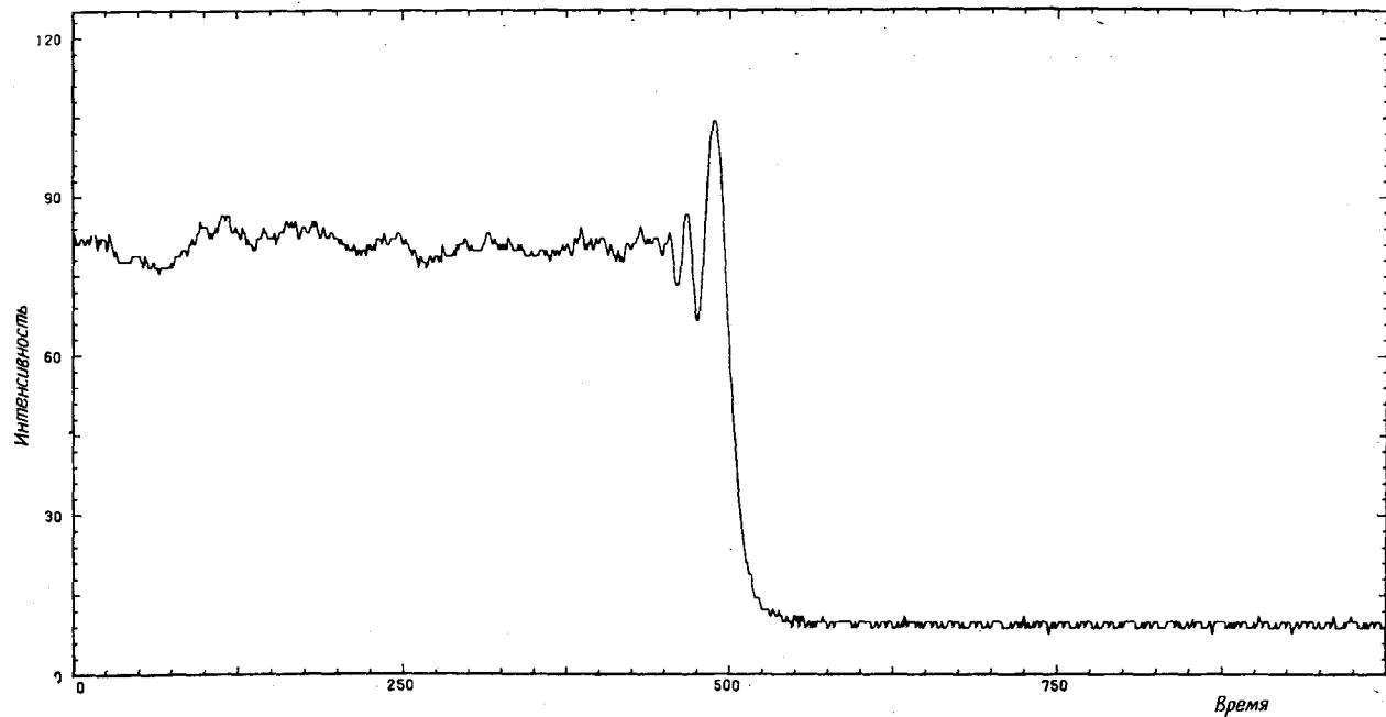
Рис. 3.16. Кривая блеска при покрытии Альциона Луной 11 сентября 1973 г. Эта кривая характерна для одиночной звезды. (Кривая получена Эвансом в Техасском университете.) По оси абсцисс отложено время в миллисекундах, по оси ординат — интенсивность в произвольном масштабе.
