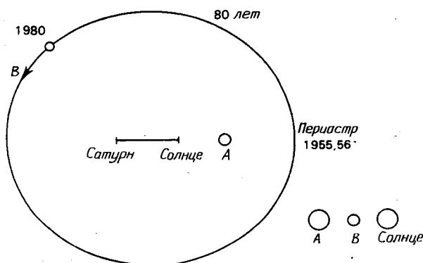
Рис. 7.1. Истинная орбита системы \alpha Центавра. Система включает третью звезду — очень удаленный от основных компонентов красный карлик. Объект A сравним с Солнцем, объект B обращается по орбите размером с орбиту Нептуна. Кружки внизу справа представляют относительные размеры компонентов пары и Солнца.
