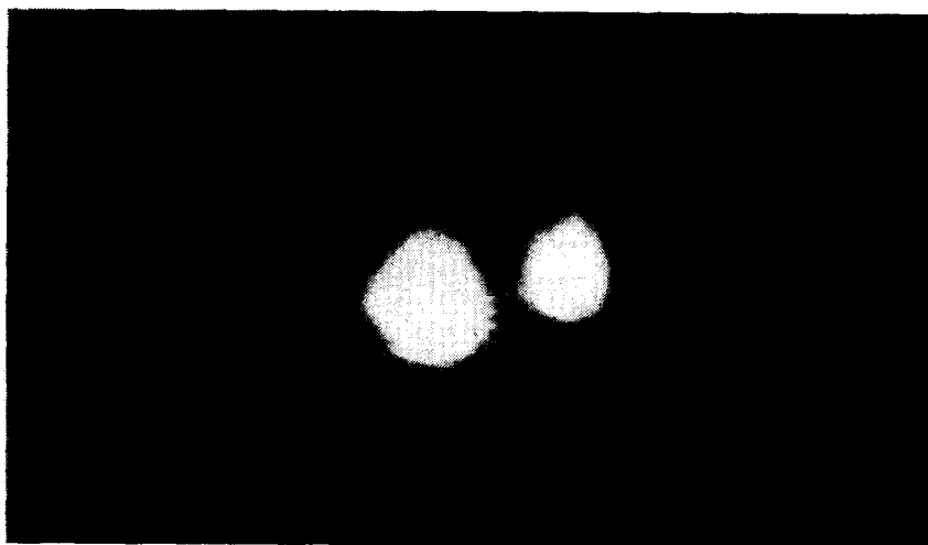
Рис. 3.11. Фотография двойной звезды \text{ADS 2799} = \text{OZ 65 } \alpha = 3^{\text{h}}47^{\text{m}}03^{\text{s}} , \delta = +25^{\circ}26' (1950). Рефрактор апертурой 50 см, экспозиция 1с 1967, 818, позиционный угол 203,9^{\circ} , разделение 0,65'' , звездная величина 6,5 и 6,8^{\text{m}} . Фокусное расстояние 22,5 м, увеличение 300 раз, расстояние между центрами изображений 72 мкм. (Фотография Фоссата, обсерватория в Ницце.)
