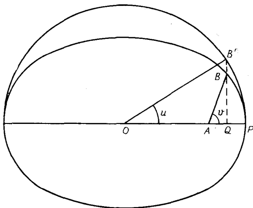
Рис. 6.1. Истинная орбита
